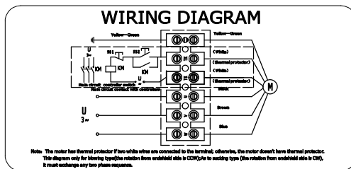
WIRING DIAGRAM (接线图) :
