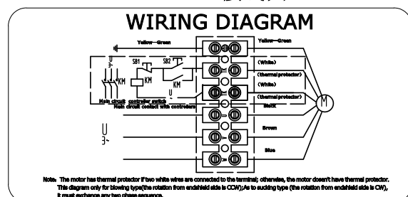
WIRING DIAGRAM (接线图) :
